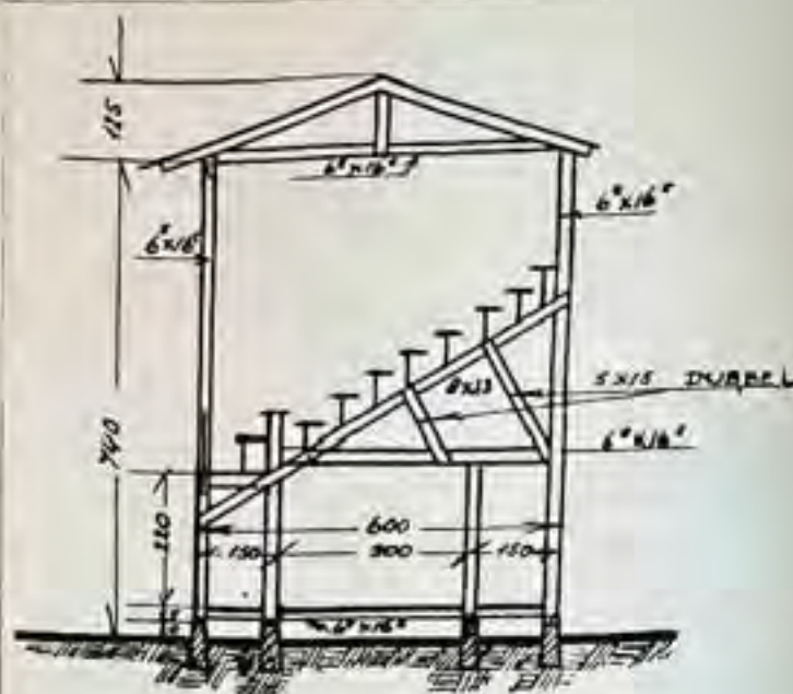
DOORSNEDE
